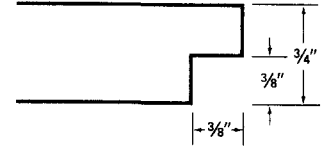
Shadow Line Edge (SL)
