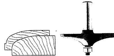
HANDRAIL/TABLE EDGE
